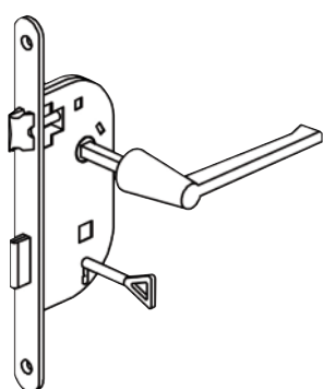
■ PÊNE DORMANT 1/2 TOUR (PDDT)
