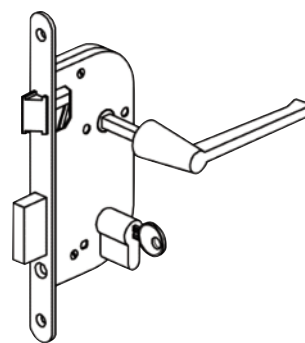
■ SERRURE DE SÛRETÉ 1 OU 3 POINTS
